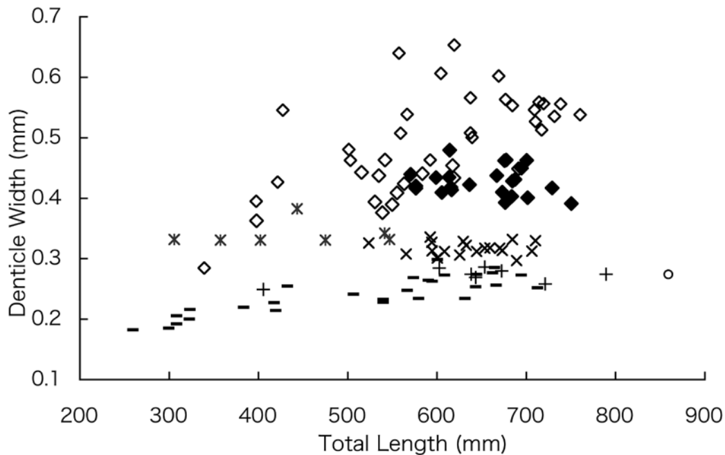
Figure 10. Width of dermal denticle. Apristurus melanoasper (◆, present specimens; ◇, North Atlantic specimens); A. gibbosus (*); A. japonicus (x); A. laurussonii (-); A. sinensis (+); A. saldanha (o).
